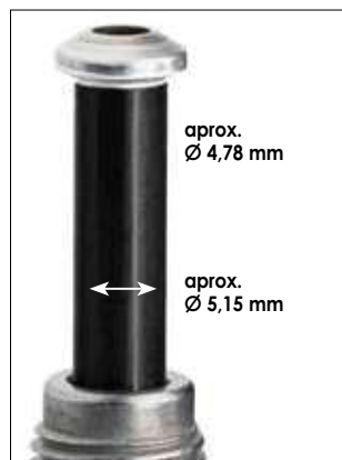
Posicionamento da tubagem para raspar o revestimento
